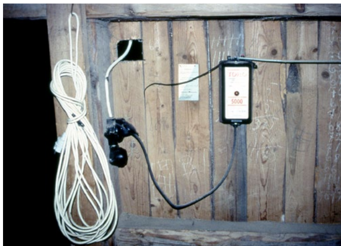
Elstängselapparat får inte placeras på en oskyddad trävägg.
